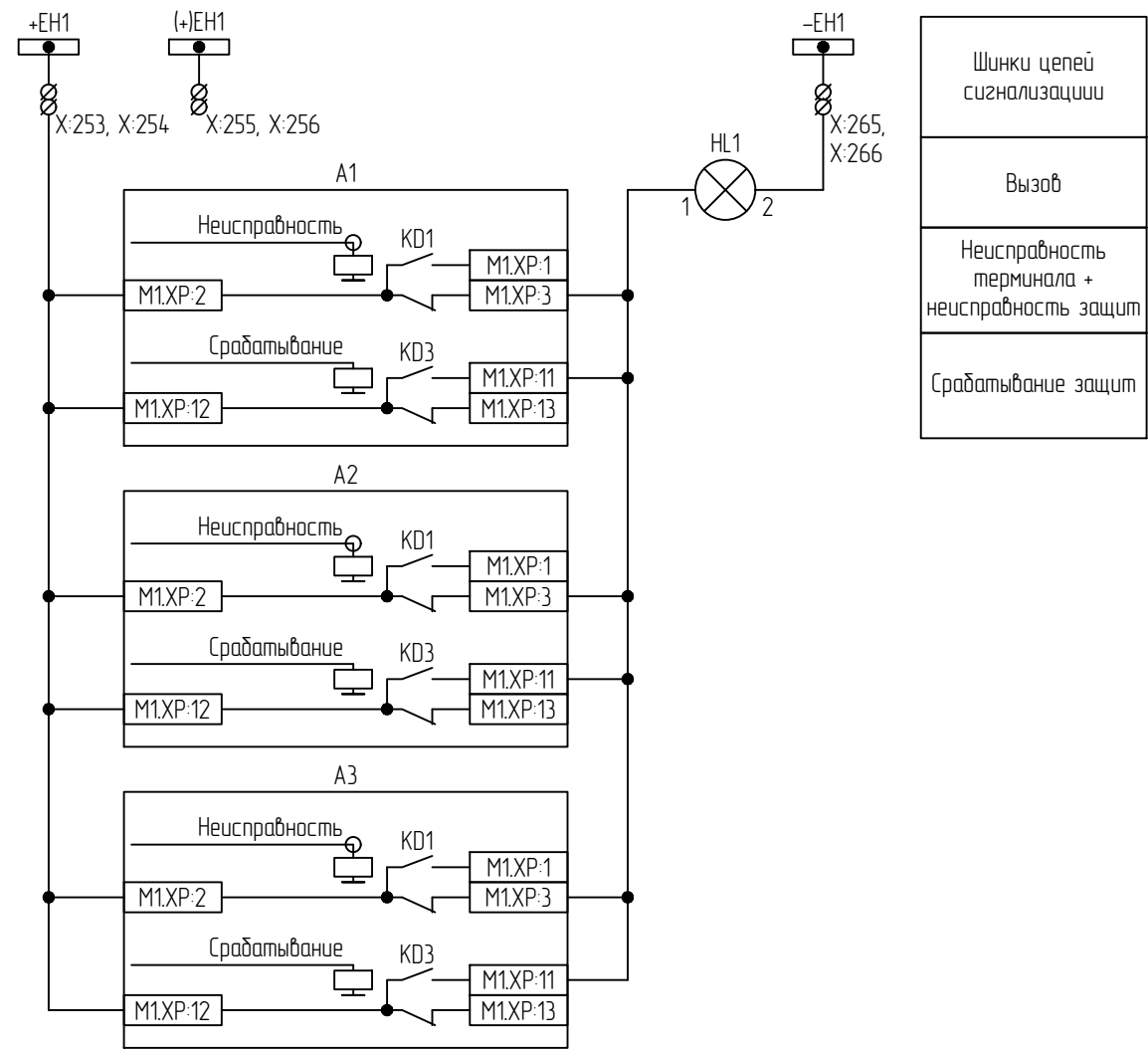
Цепи РАС
