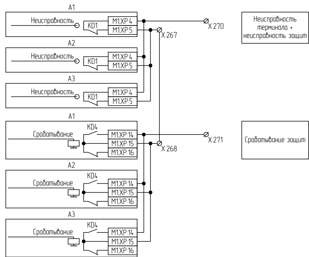
Цепи РАС
